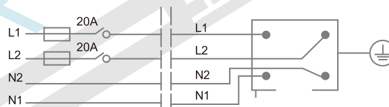
四線二迴路導軌系統
