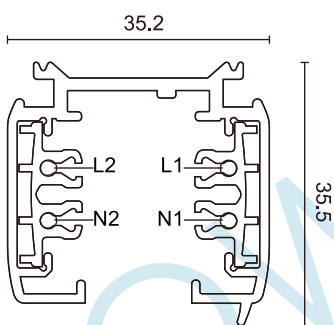
產品尺寸 (mm)
