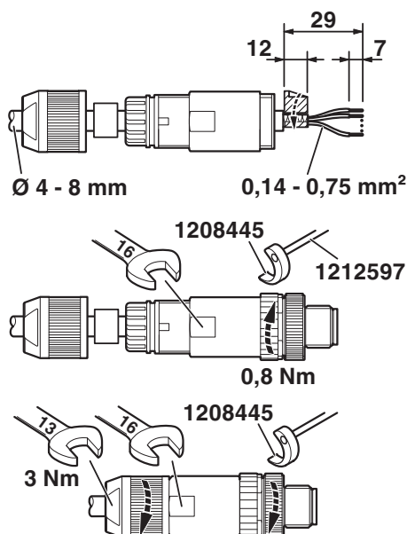
Funktionszeichnung
