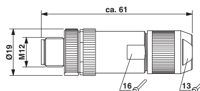
Stecker M12-SPEEDCON, gerade, geschirmt
