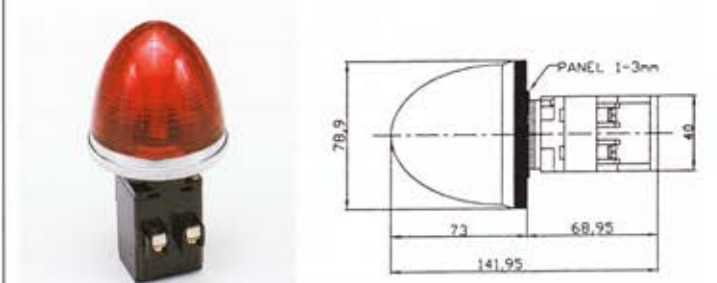
FPLB-30 30 φ 閃爍型特大圓指示燈
