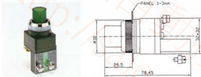
LPBN2511 25 \phi 直接式照光按鈕
