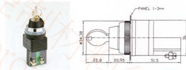
KSS3012 30 φ 鑰匙開關
