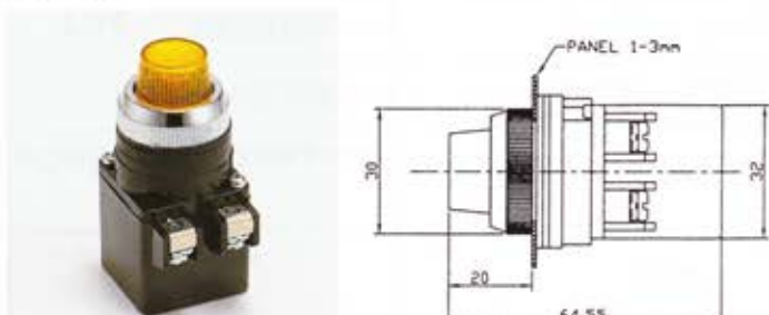
PLF-25 25 φ 平圓形指示燈
