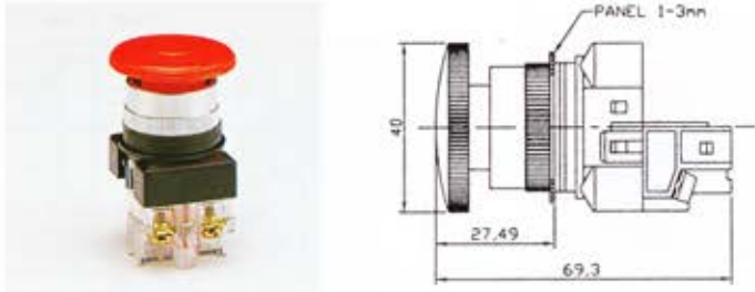
EPBK2511 25φ 大頭按鈕
