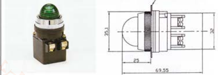
PLR-30 Round lens, PLF-30 Flat round lens 30 φ 圓形指示燈 ; 30 φ 平圓形指示燈
