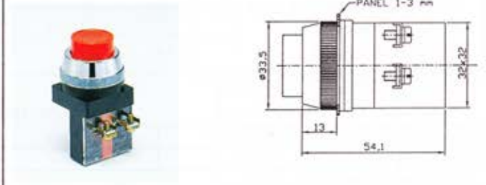
PBL3011 30 φ 凸頭按鈕
