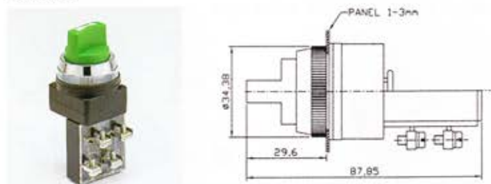
SS3013 30 φ 短柄選擇開關
