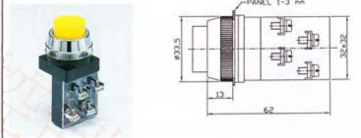
PBR-3011 30 φ 平頭按鈕加防水帽
