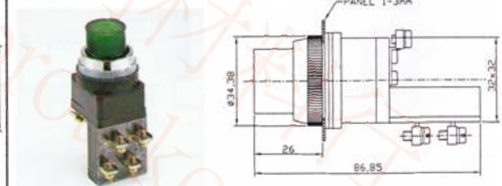
LPBT3011 30 \phi 變壓器式照光按鈕
