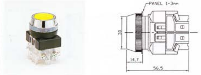
PBK3011 30φ 平頭按鈕
