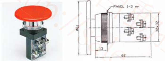
EPBLR3011 30φ 特大頭護圈按鈕
