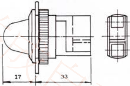
NPLF-25A 25φ 平頭型指示燈
