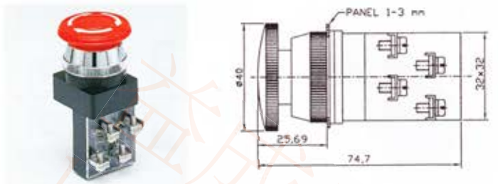
EPBL3011 30φ 特大頭按鈕
