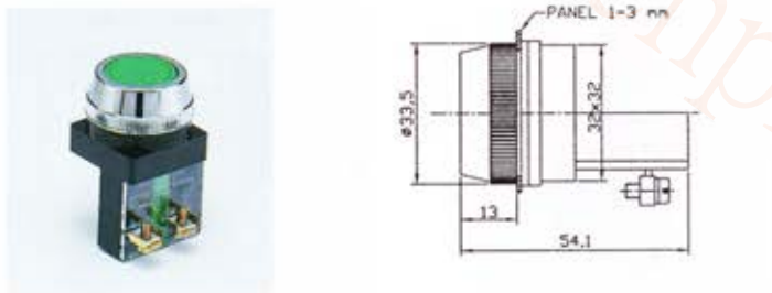
PB30-1b 30 φ 平頭按鈕
