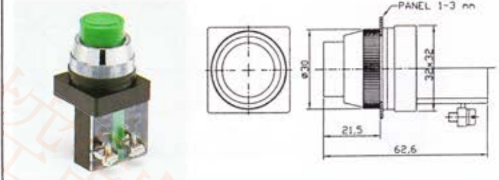
PBL25-1b 25 \phi 凸頭按鈕
