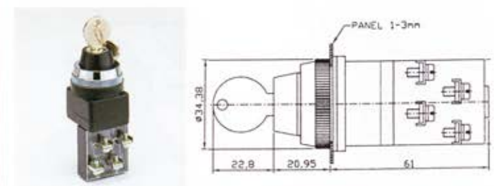
KSS3013 30 φ 鑰匙開關
