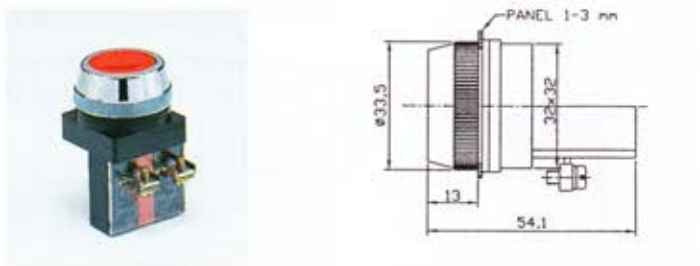
PB3011 30 φ 平頭按鈕
