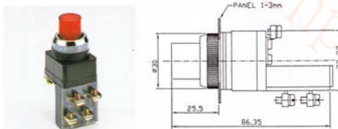
LPBT2511 25 \phi 變壓器式照光按鈕
