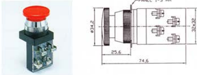
LEPB25-1b 25 φ 急停按鈕
