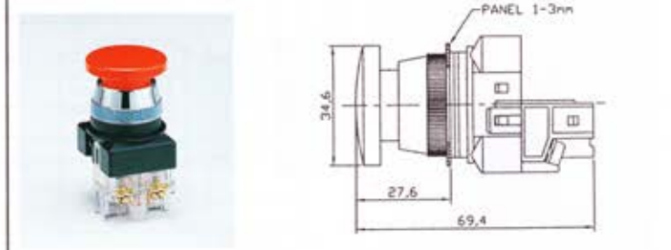
EPBK 2211 22φ 大頭按鈕
