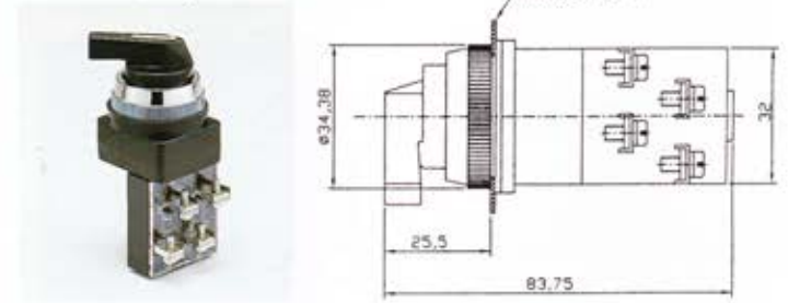
LSS3013, 3 position 30 φ 長柄選擇開關
