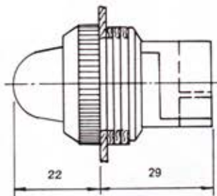
NPLF-25B 25φ 平圓形指示燈
