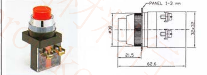
PBL25-11 25 \phi 凸頭按鈕
