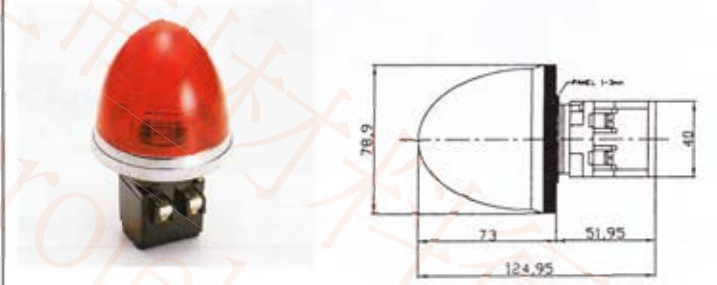
PLB-30 30 φ 特大圓形指示燈
