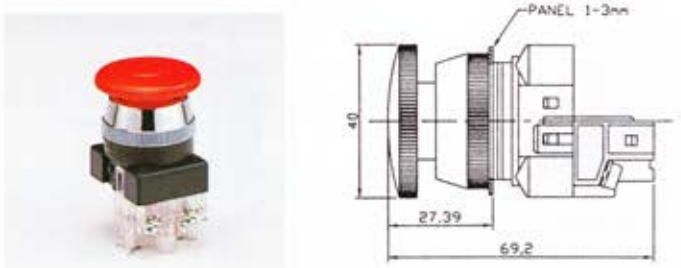
EPBK3011 30φ 大頭按鈕
