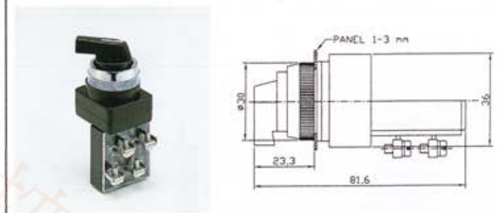
LSS2513 25 \phi 長柄選擇開關
