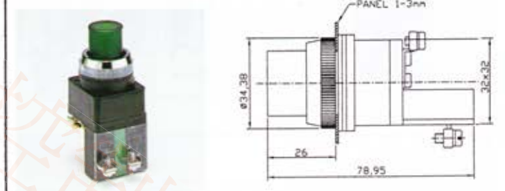
LPBN3011 30 \phi 直接式照光按鈕
