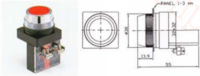
PB2511 25 \phi 平頭按鈕
