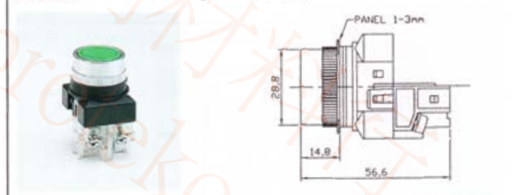
PBK25-1b 25φ 平頭按鈕
