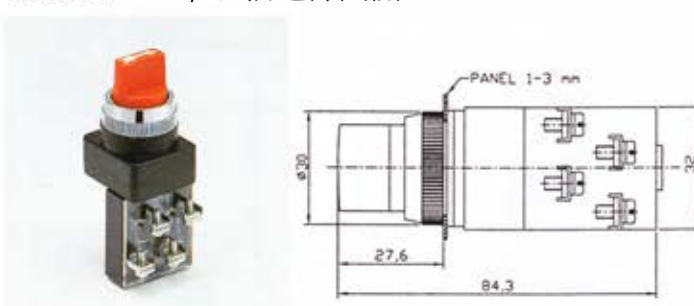
SS2513 25 \phi 短柄選擇開關
