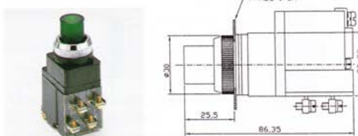
LPBTG2511 25 \phi 護圈照光按鈕
