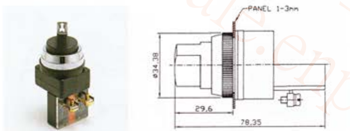
SS30-1b 30 φ 短柄選擇開關
