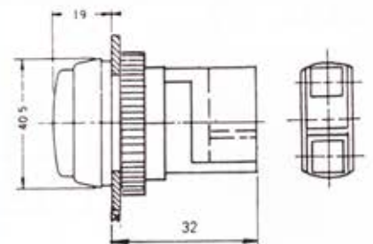
NPLS-30A 30φ 方形指示燈
