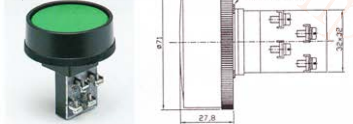
PBK22-1a Mounting hole 22φ 平頭按鈕
