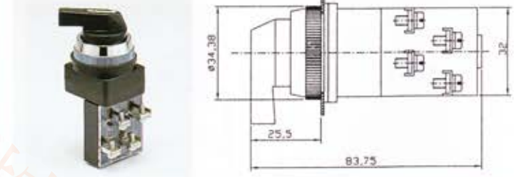
KSS30-1a 30 φ 鑰匙開關
