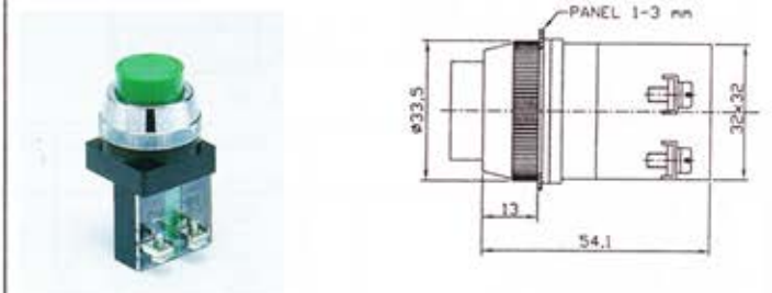
PBL30-1b 30 φ 凸頭按鈕
