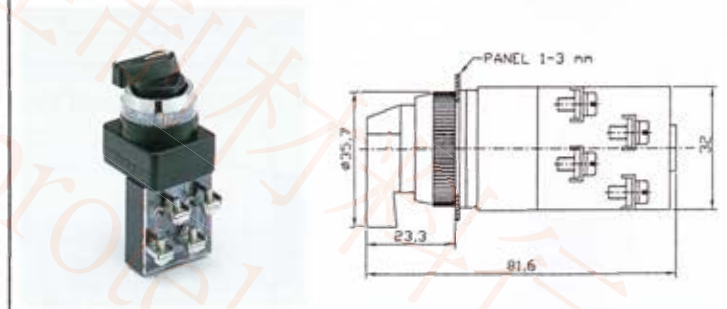
KSS25-1a 25 \phi 鑰匙開關
