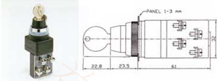
SS30-1a 30 φ 短柄選擇開關
