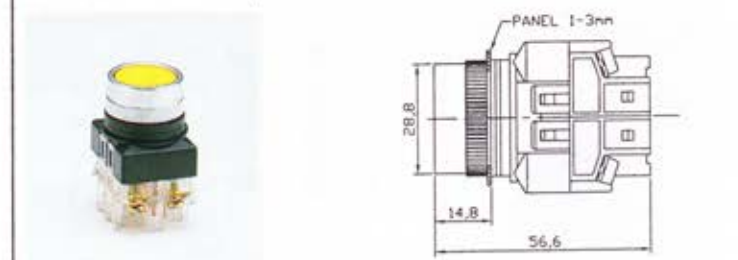
PBK2511 25φ 平頭按鈕
