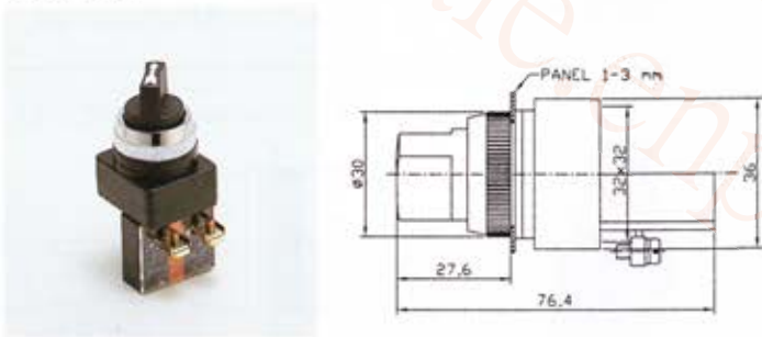
SS2512 25 \phi 短柄選擇開關
