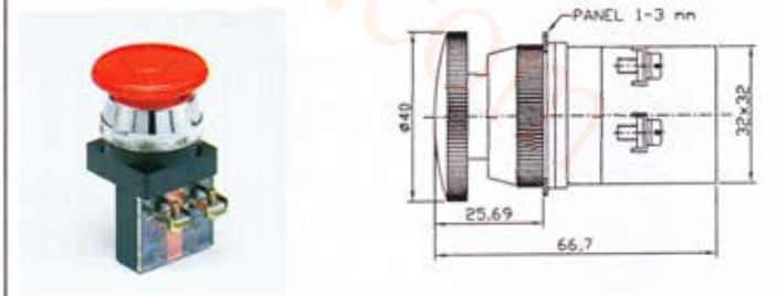
EPB3011 30 φ 大頭按鈕
