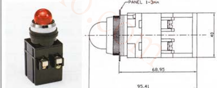
FPL-30 30 φ 閃爍型平圓指示燈
