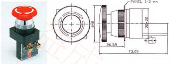
LEPB2511 25 φ 急停按鈕
