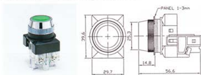
PBK22-1a Mounting hole 22φ 平頭按鈕
