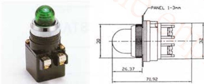
PLR-25 25 φ 圓形指示燈
