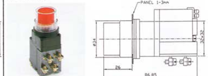
LPBTG3011 30 \phi 護圈照光按鈕
