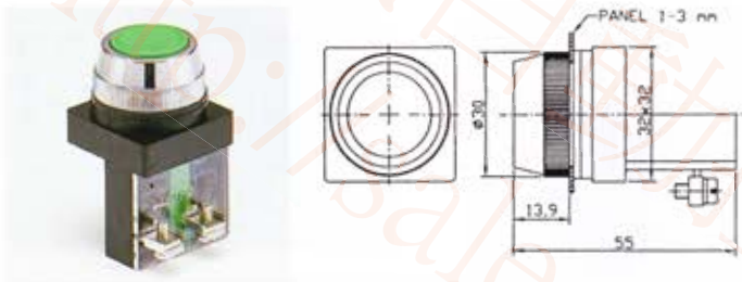
PB25-1b 25 \phi 平頭按鈕
