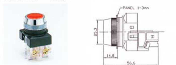
PBK22-1b 22φ 平頭按鈕
