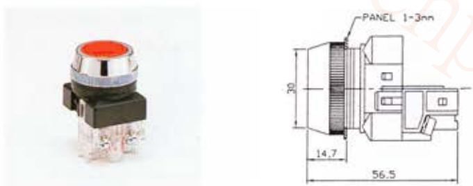
EPBK30-1b 30φ 大頭按鈕
