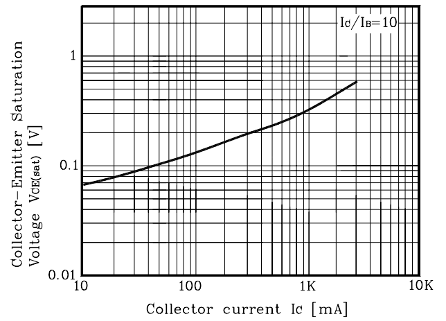
Fig. 2 V_{CE(sat)} - I_C
