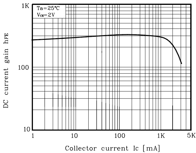
Fig. 3 h_{FE} - I_C
