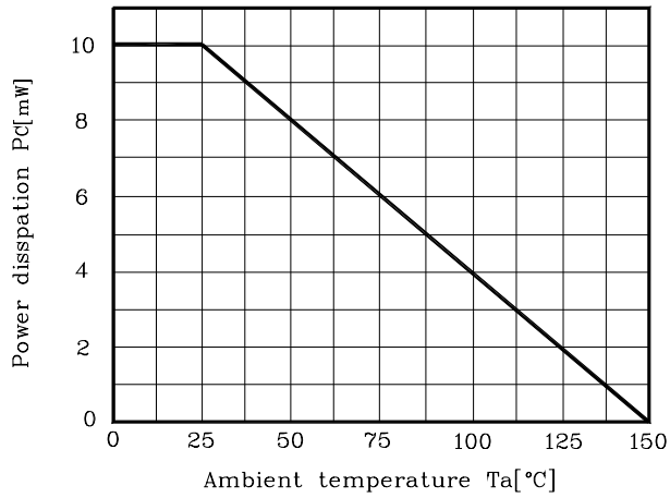
Fig. 1 P_C - T_a
